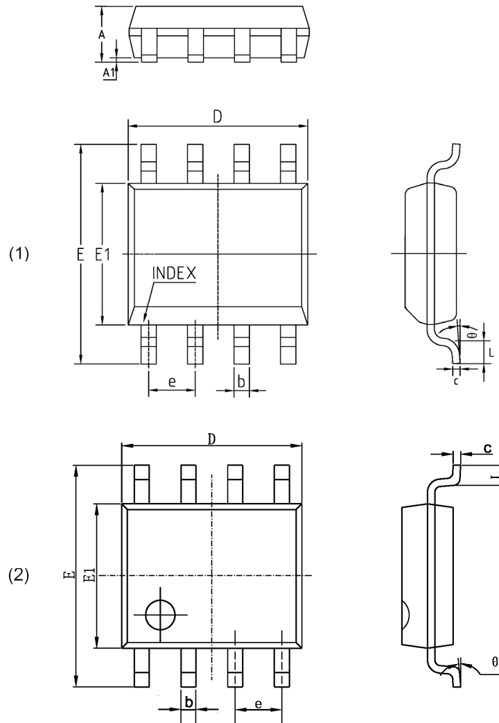
SOP 8
